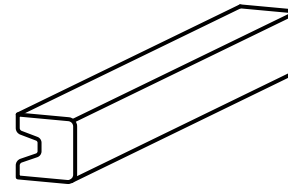
Mini Box Cap ST-MBC1 Group B Corners: DA, UA, OC 1" H x 6" L x 7/8" D
